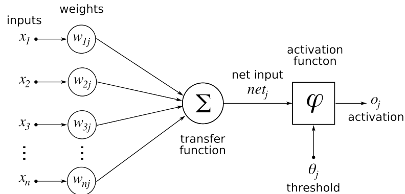
FIGURE 2.1 – Schéma d'un réseau de neurones. Ici, la fonction d'activation et la fonction de transfert sont détaillées.
