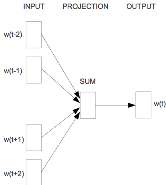
FIGURE 2.3 – Architecture CBOW du word2vec. On remarque les différents mots w en entrée entourant la position courante.
