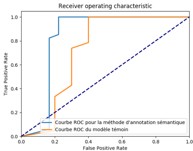
FIGURE 5.2 – Courbes ROC obtenues sur les données testées.
