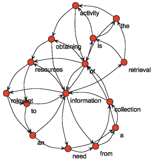
FIGURE 2.5 – Représentation de l'exemple 2.6
