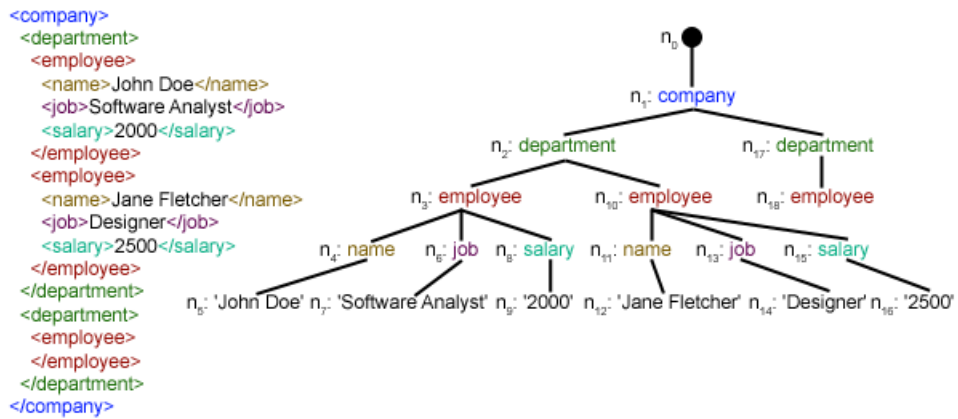
FIGURE B.1 – Liens entre Graphes et XML.
