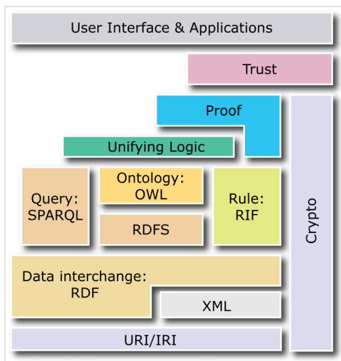
Figure 1 : Le « layer cake » du Web Sémantique 10
