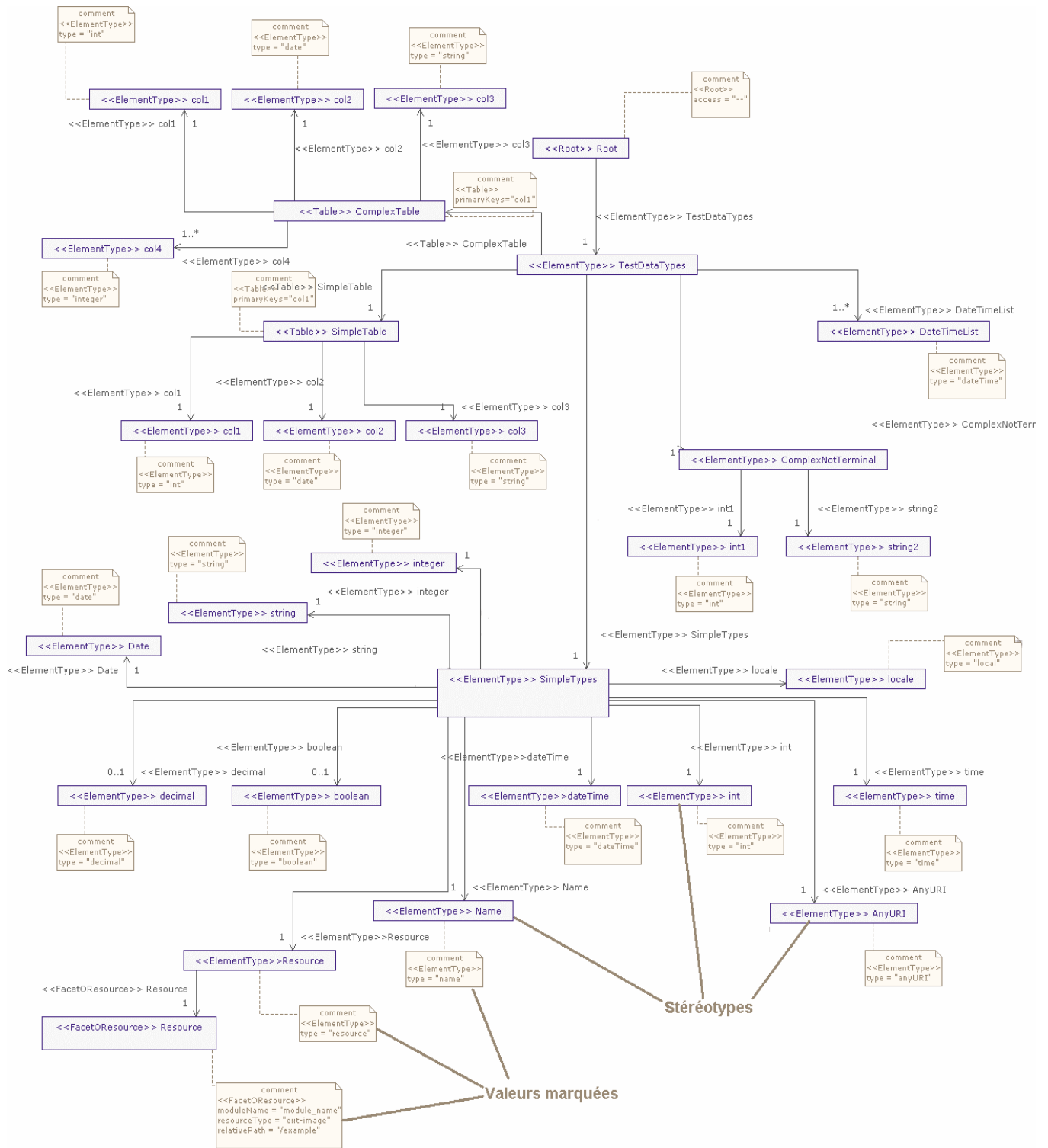
Figure 29 – Diagramme UML définissant un modèle d'adaptation
