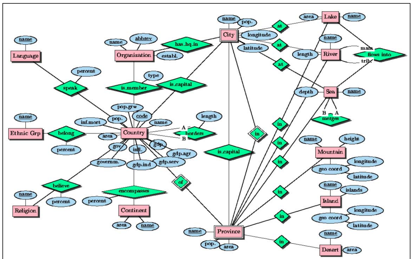
Figure 45 – Schéma entités-relations de la base Mondial définie par McBrien
